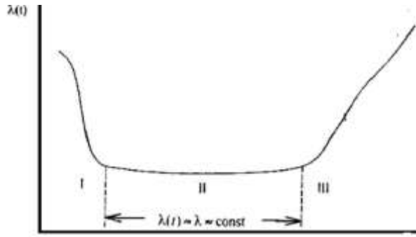
Рисунок 1. Интенсивность отказов во времени
